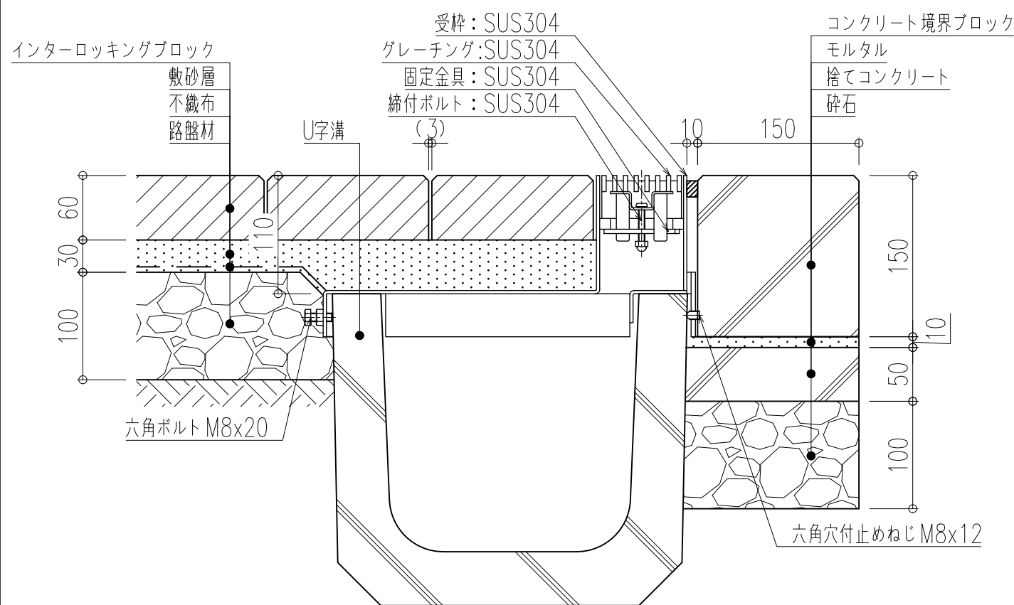
施工参考図
